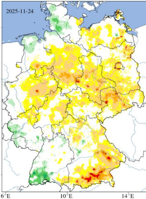
Verlauf der langjährigen Einordnung - Gesamtboden
