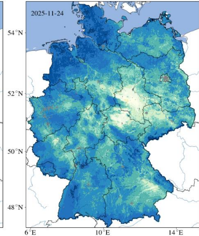
Verlauf des pflanzenverfügbaren Wassers im Oberboden
