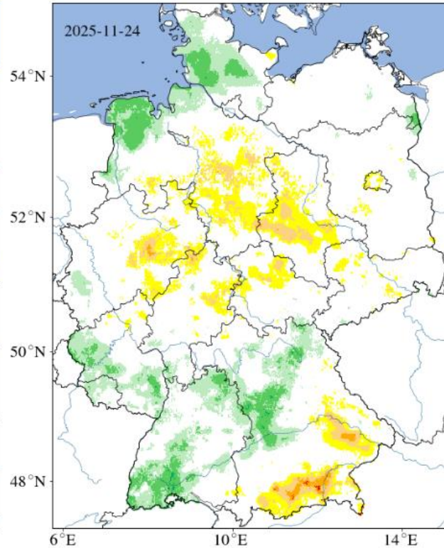
Verlauf der langjährigen Einordnung - Oberboden
