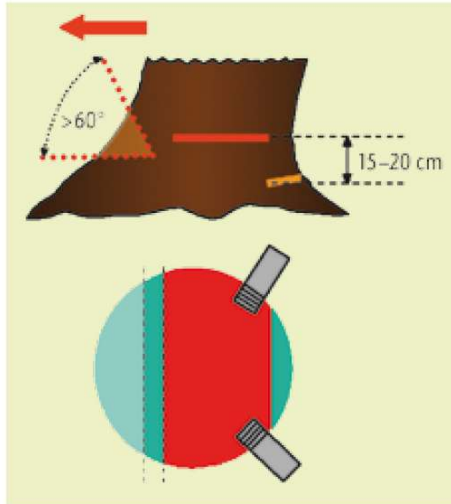
Abb. 8: Modifizierte Schnitttechnik für Laubholz mit Trockenkronen
